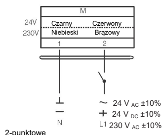
Schemat połączeń NECA...06/10 (S1) Zasilanie 24 V AC/DC / 230 V AC
