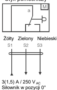
Schemat połączeń NECA...06/10 (S1) Styk pomocniczy
