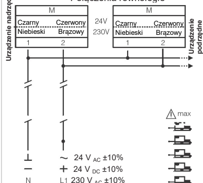
Schemat połączeń NECA...06/10 (S1) Połączenia równoległe
