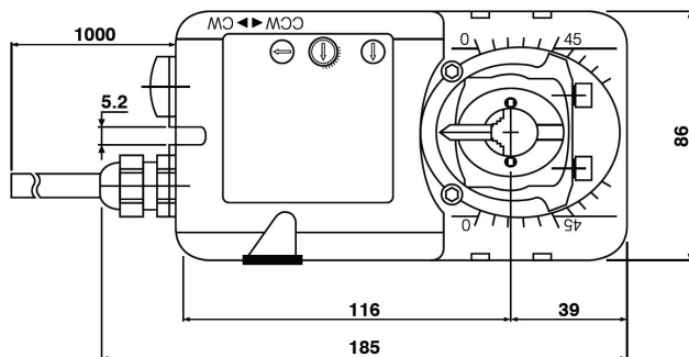
WYMIARY SIŁOWNIKA [mm]
