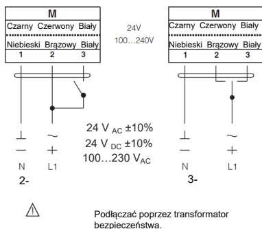
Schemat połączeń NCCA...02 Zasilanie 24 V AC / DC
