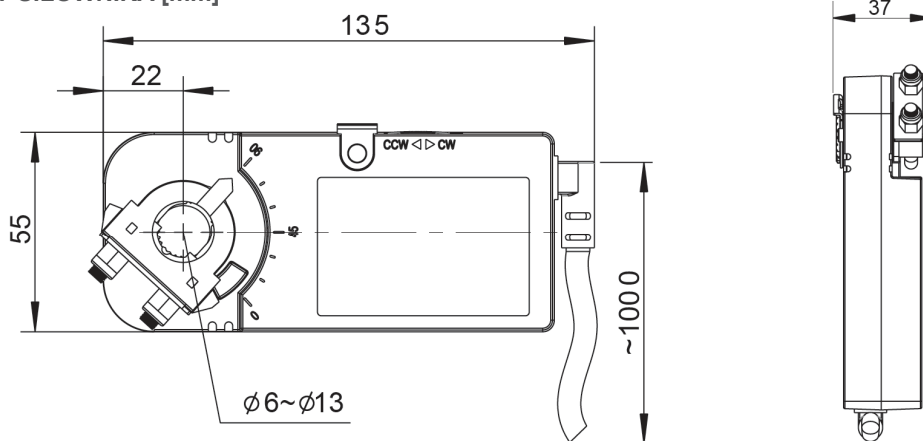
WYMIARY SIŁOWNIKA [mm]
