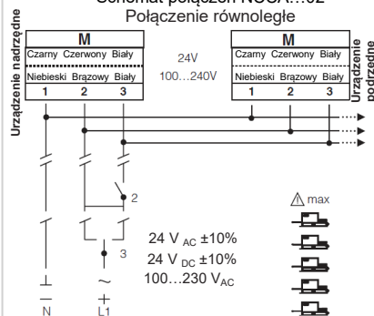
Schemat połączeń NCCA...02 Połączenie równoległe
