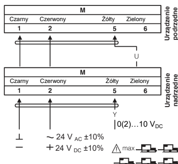
Schemat połączeń NCCM...02 Połączenie równoległe
