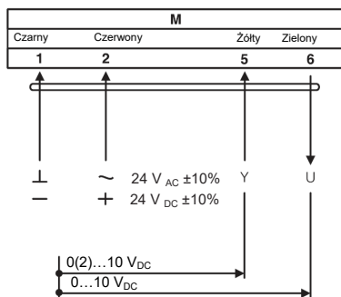
Schemat połączeń NCCM...02 Zasilanie 24 V AC / DC
