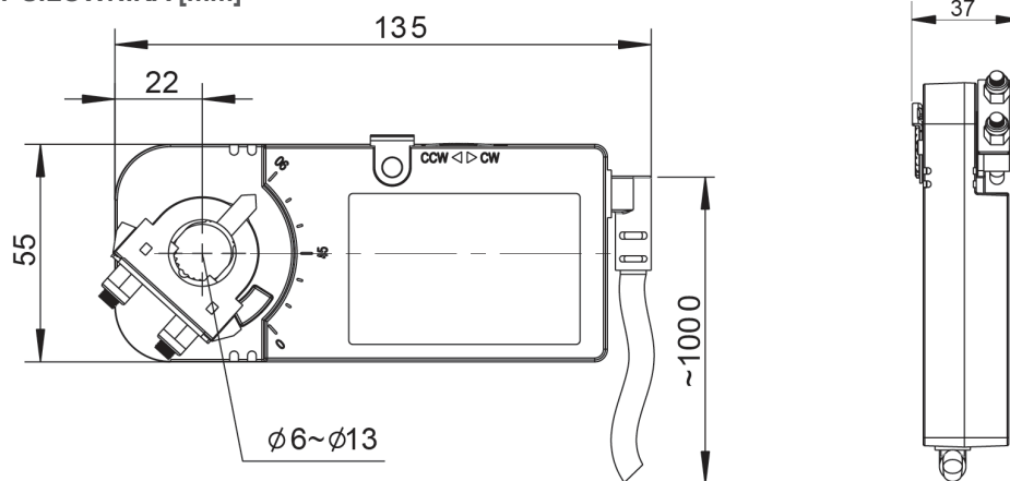
WYMIARY SIŁOWNIKA [mm]
